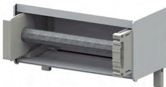
Figura 44. Sistema de testeros que posibilitan extracción del eje
